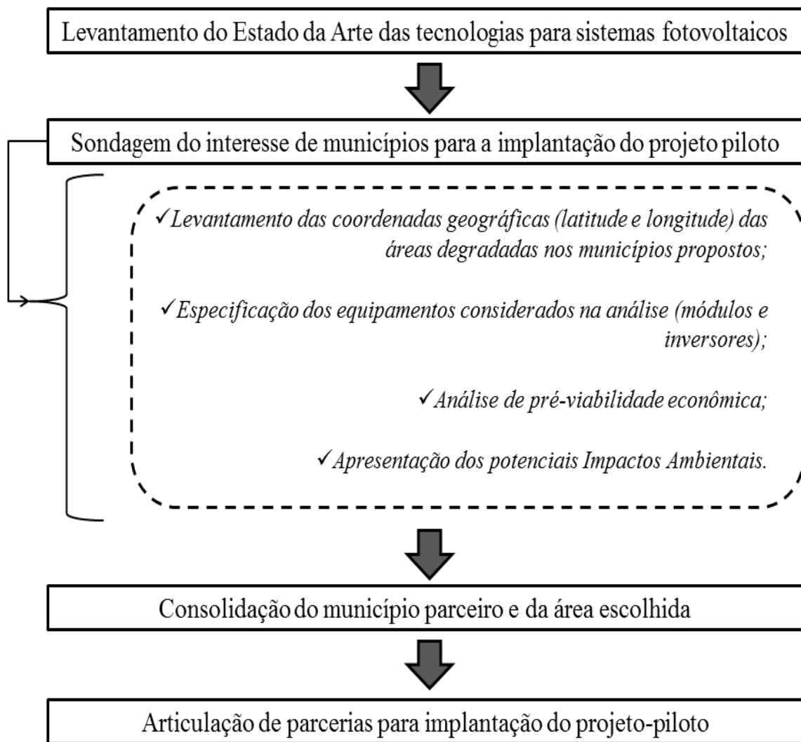
Figura 3: Fluxograma metodológico do projeto Fonte: Elaborado pelo autor.
