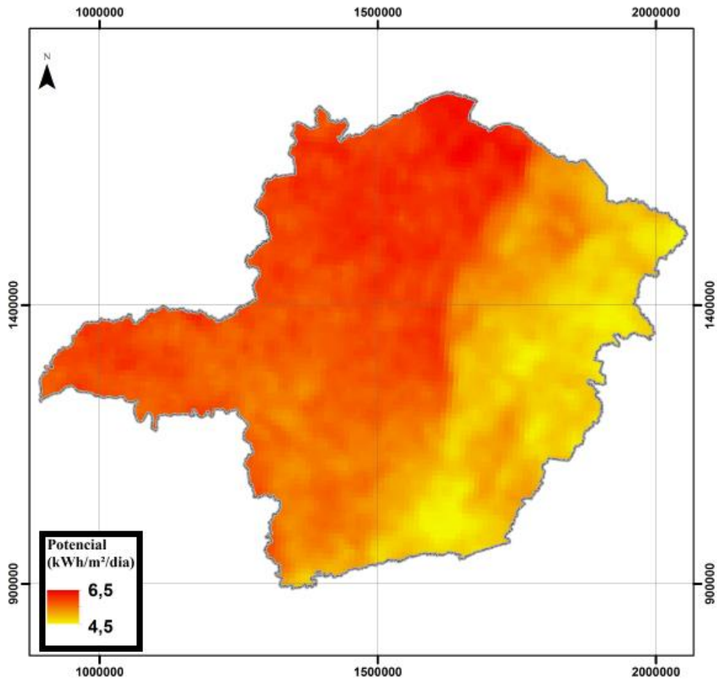
Figura 2: Radiação solar média diária anual em Minas Gerais Fonte: (SILVA, 2014).
